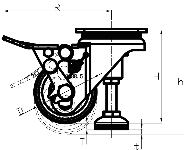
支撐升降腳輪 Levelling Caster
